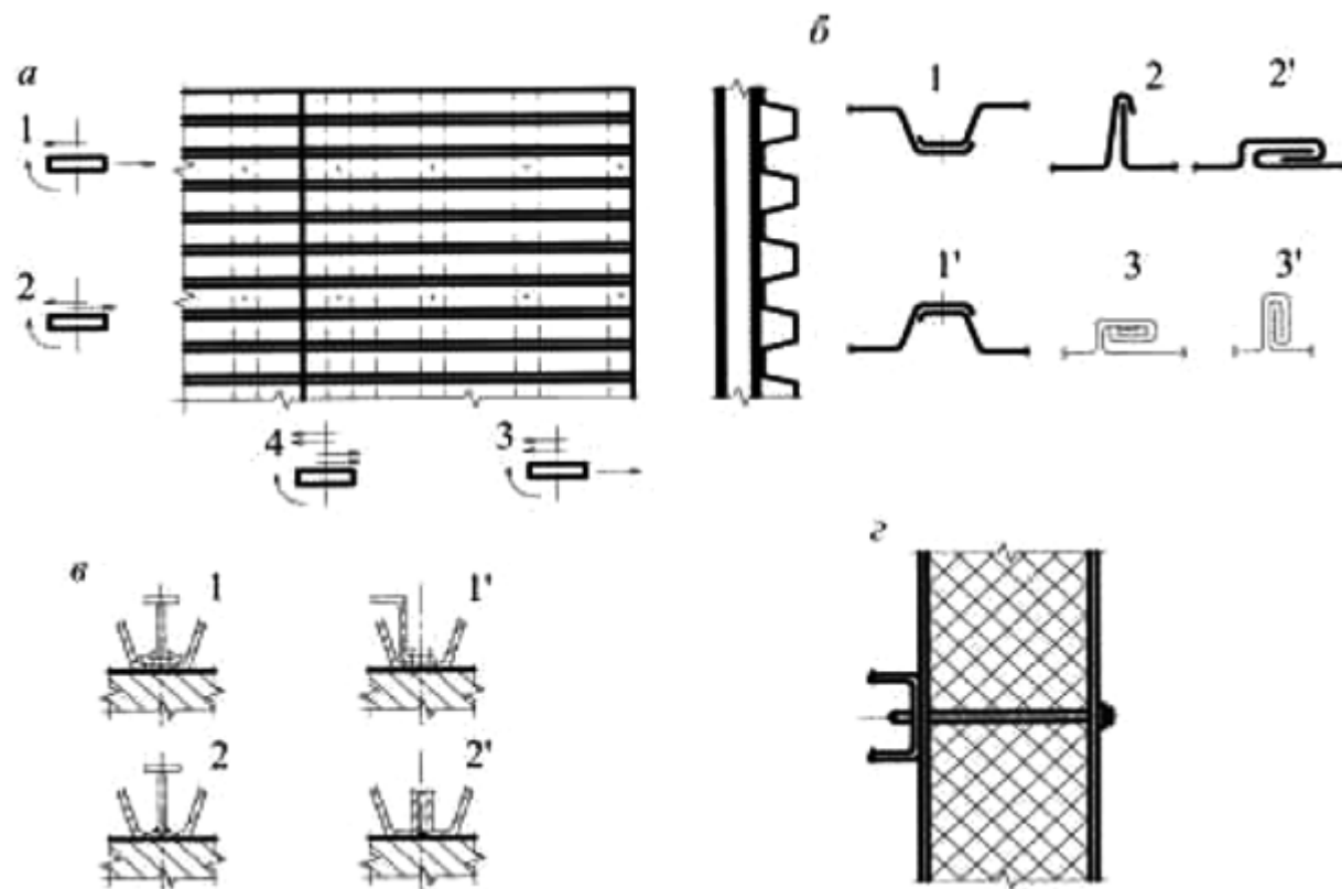
а - фрагмент конструкции покрытия со стальным профилированным настилом и схема действия сил на опорах (1 - соединения в среднем участке; 2
